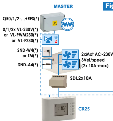
(*) Accessori/es: SND-A4, SND-W4, TM, SDI.2x10A, VL..., QR0/1/2-230(400)+RES
