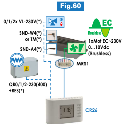
(*) Accessori/es: SND-A4, SND-W4, TM, VL-230V, QRO/1/2-230(400)+RES
