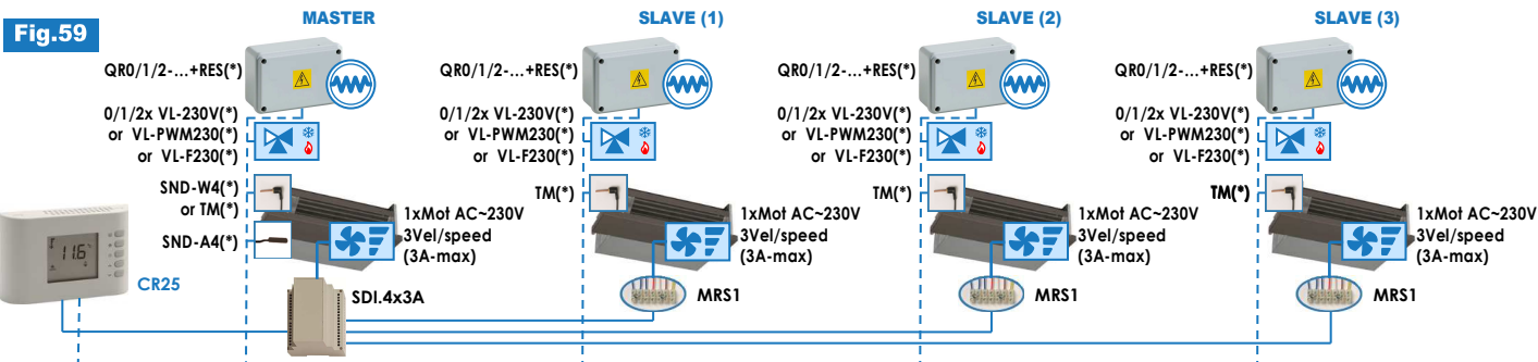
(*) Accessori/es: SND-A4, SND-W4, TM, VL..., QR0/1/2-230(400)+RES, SDI.4x3A
