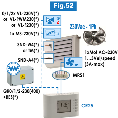
(*) Accessori/es: SND-A4, SND-W4, TM, VL..., QR0/1/2-230(400)+RES, MS-230V
