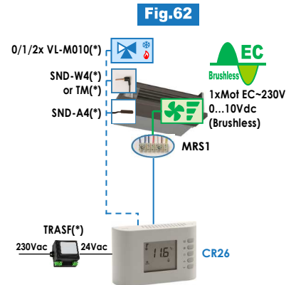
(*) Accessori/es: SND-A4, SND-W4, TM, VL-M010
