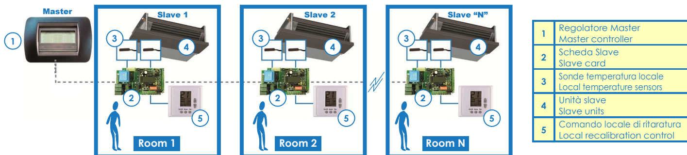
Master-Slave per la Regolazione di Zona con parametri ritarabili Master-Slave for the Regulation of Area with recalibrated parameters
