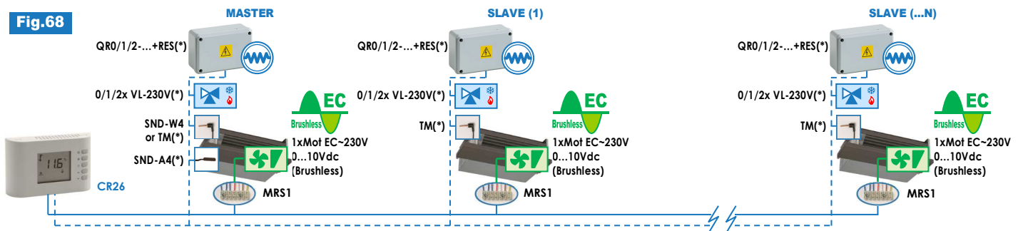
(*) Accessori/es: SND-A4, SND-W4, TM, VL..., QRO/1/2-230(400)+RES
