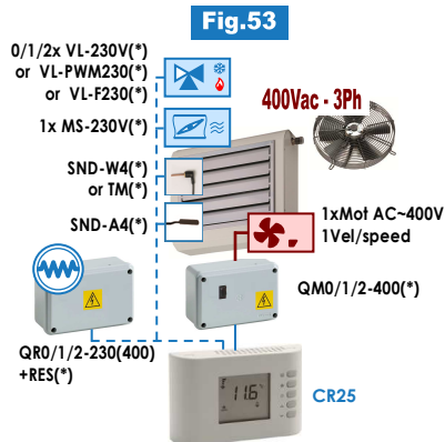
(*) Accessori/es: QM0/1/2-400, SND-A4, SND-W4, TM, VL..., QR0/1/2-230(400)+RES, MS-230V
