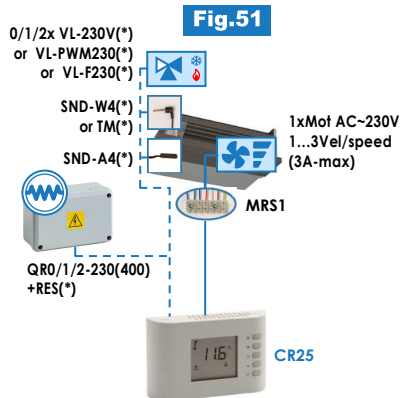
(*) Accessori/es: SND-A4, SND-W4, TM, VL..., QR0/1/2-230(400)+RES
