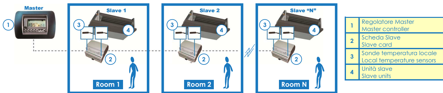
MASTER-SLAVE per la Regolazione di Zona con SET-POINT fisso MASTER-SLAVE for the Regulation of the Area at fixed SET-POINT
